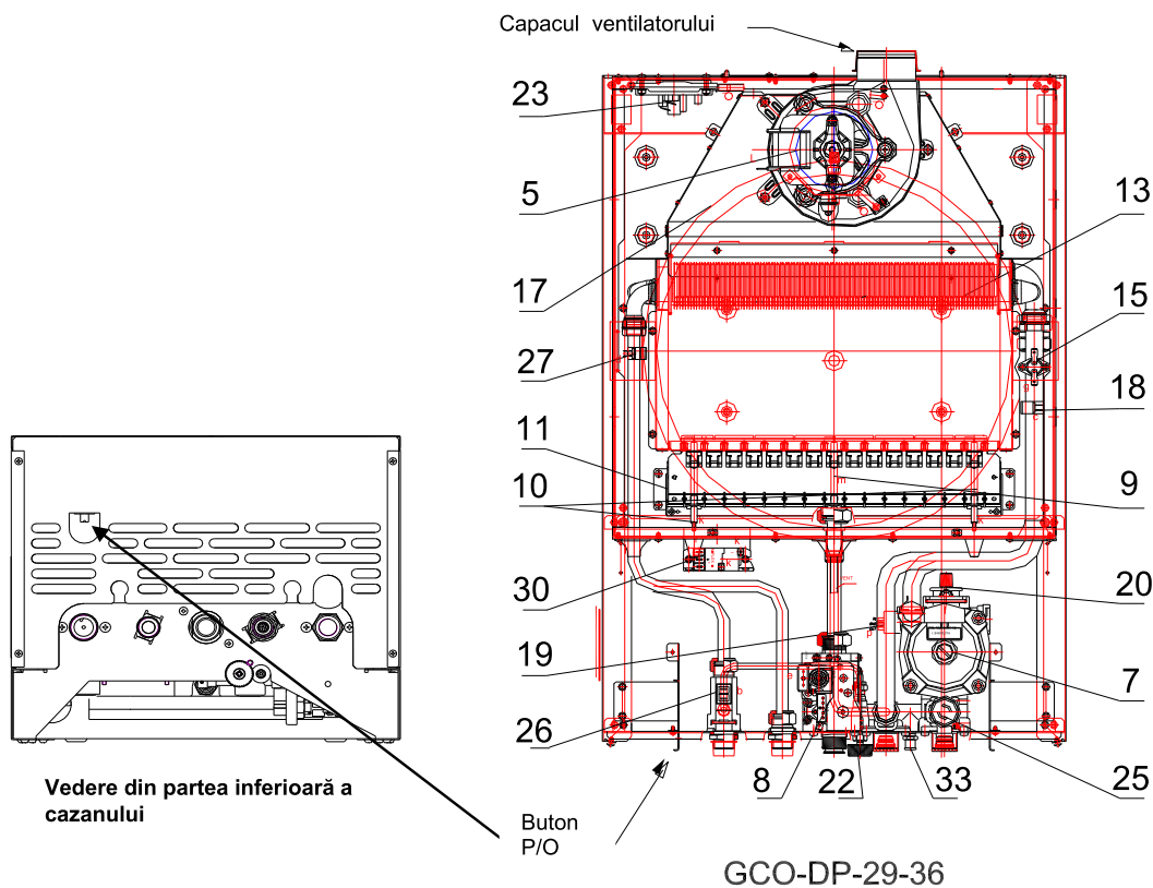
Fig. 2.2.1.2 Părțile componente ale microcentralei MaxiTerm
