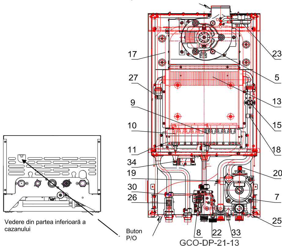
Fig. 2.2.1.1 Părțile componente ale microcentralei MINITERM
