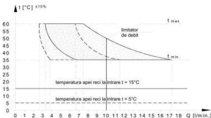
Fig. 2.4.2.1. Diagrama - temperatura ACM în funcție de debit la microcentralele GCO-DP-21-13-24/24
