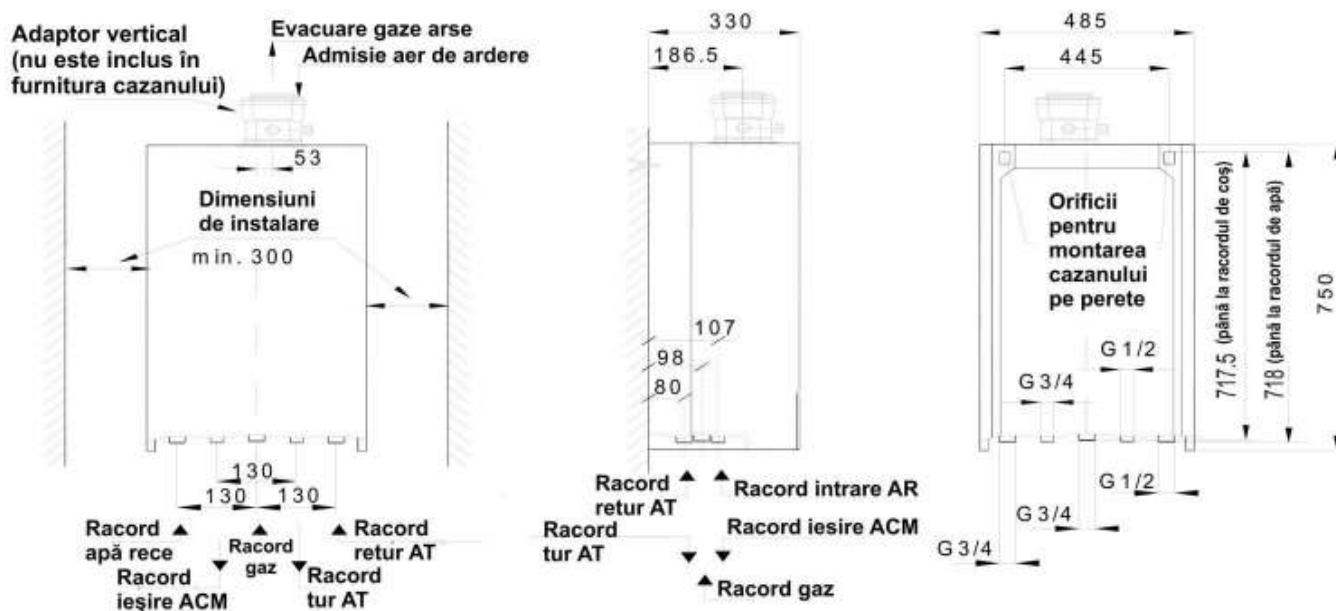
Fig. 3.3.2 Dimensiuni de instalare pentru cazanele MaxiTerm GCO-DP-29-36
