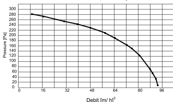
Fig. 3.7.3.1. Grafic pentru caracteristica ventilatorului
