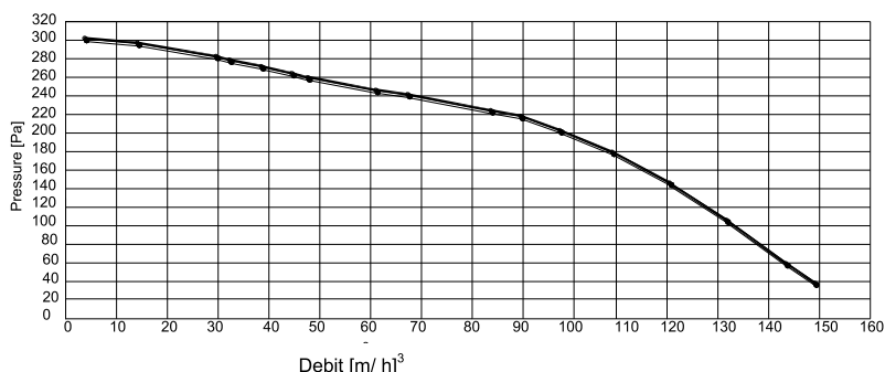
Fig. 3.7.3.1. Grafic pentru caracteristica ventilatorului
