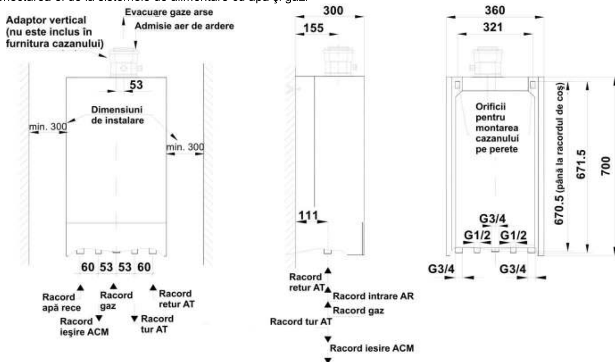
Fig. 3.3.1 Dimensiuni de instalare pentru cazanele MiniTerm GCO-DP-21-13
