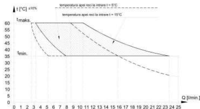
Fig. 2.4.2.2. Diagrama - temperatura ACM în funcție de debit la microcentralele GCO-DP-29-36-35/35
