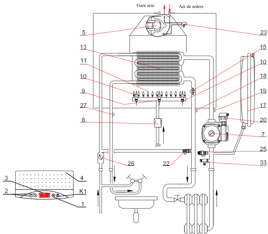
Fig. 2.2.1.3 Diagrama de funcționare a microcentralei
