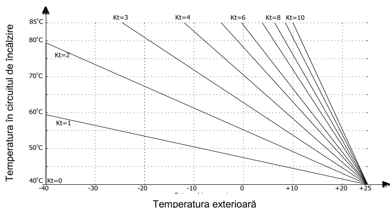
Fig. 2.4.1.1.1. Curba de încălzire
